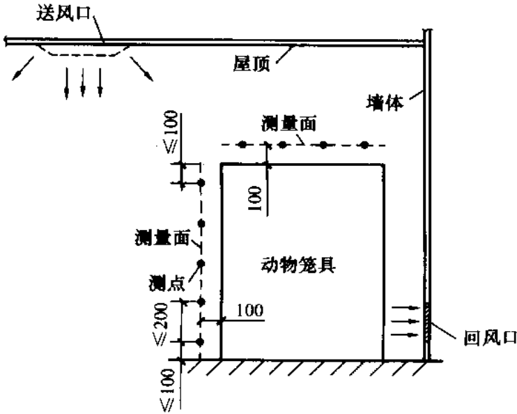
图 10.1.6 测点布置
